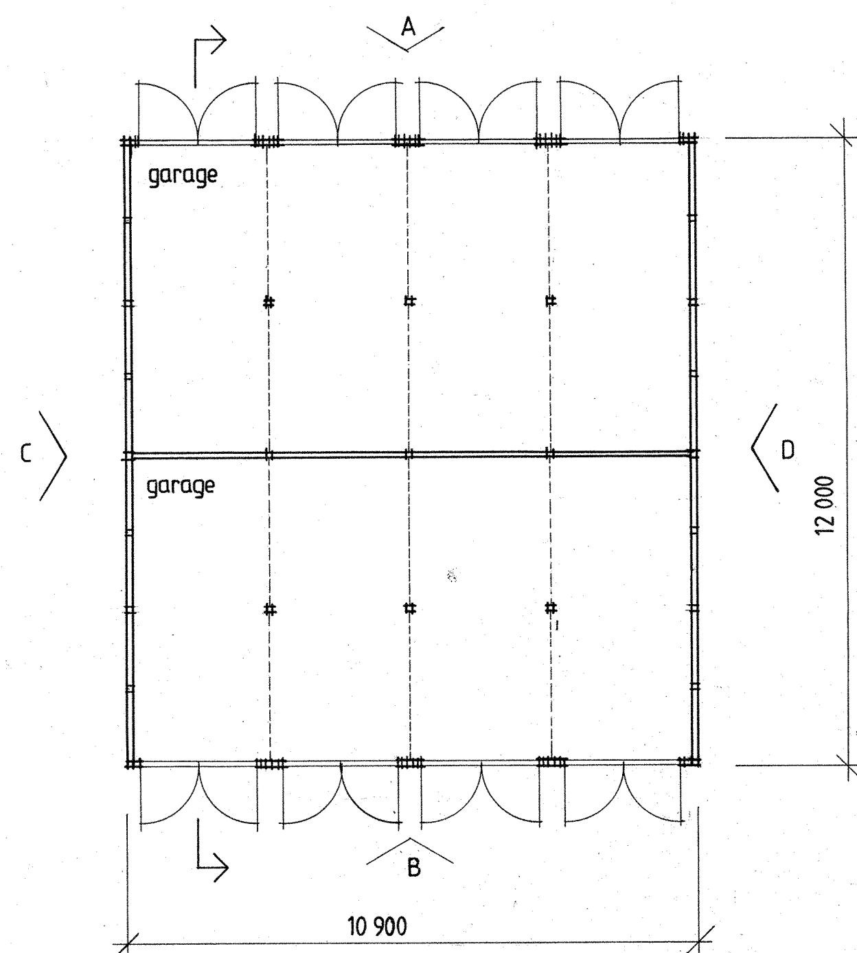
GARAGE G1 o. G4
